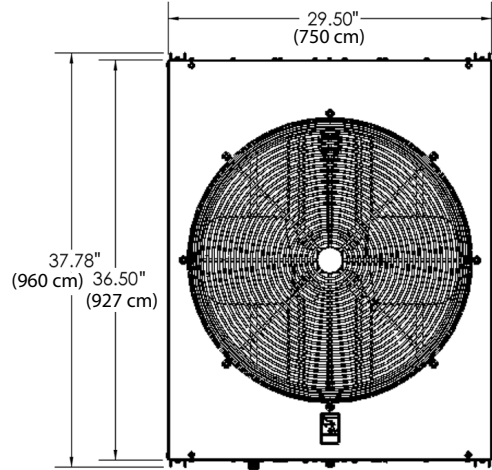
TOP VIEW--VRC5061B
